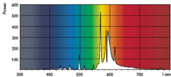
MASTER Agro Agro 400W
